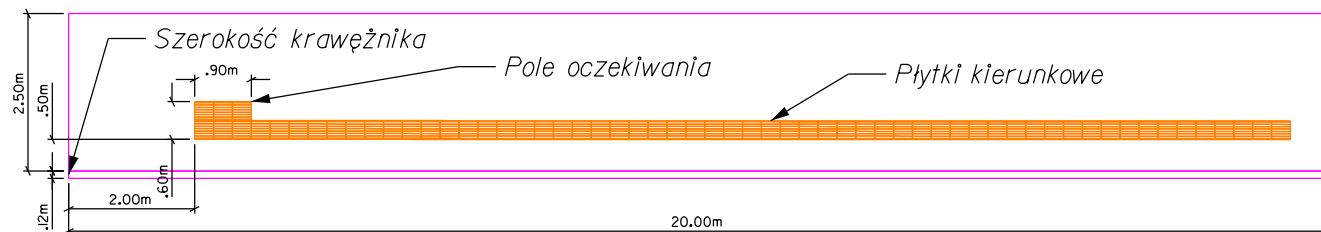
Peron autobusowy o minimalnej długości 20m
